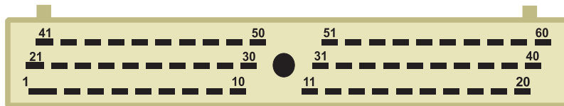
Conector de 60 vias
