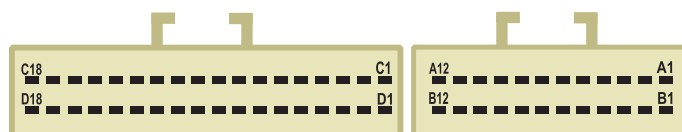
Conector de 24+36 vias
