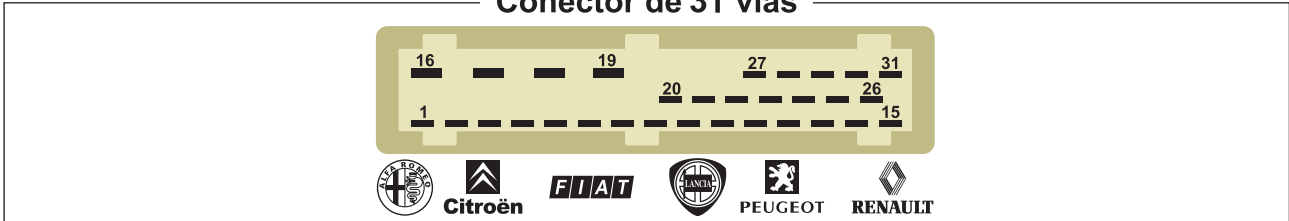
Conector de 31 vias
