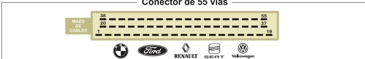
Conector de 55 vias
