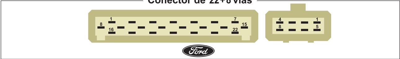
Conector de 22+8 vias
