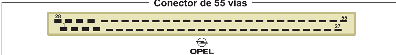
Conector de 55 vias
