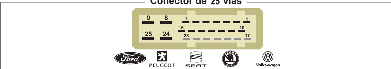
Conector de 25 vias
